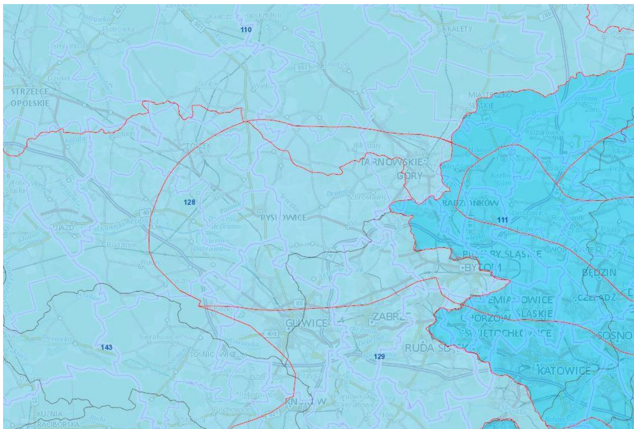
Ryc. 3 Rozmieszczenie JCWPd
