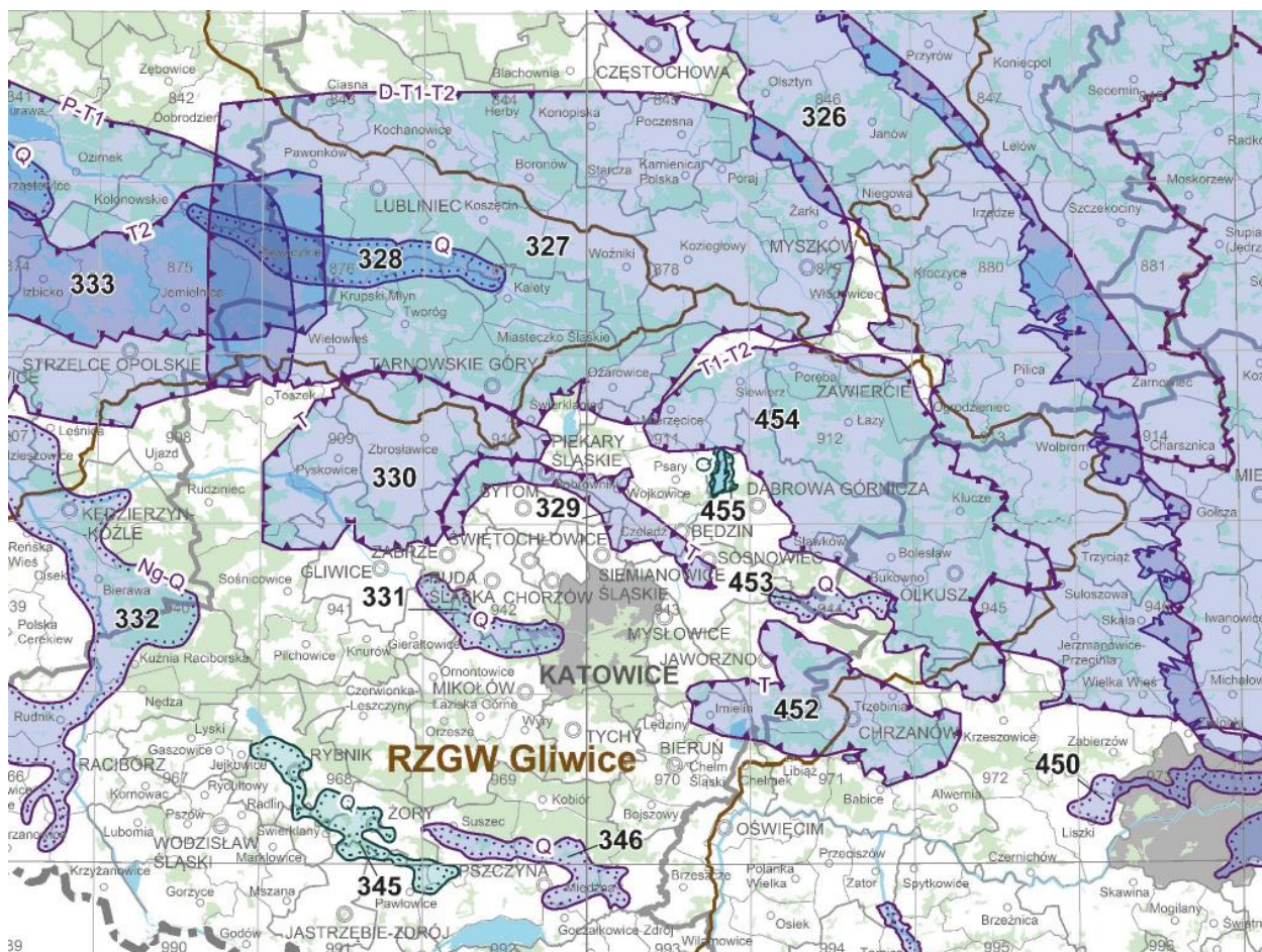
Ryc. 2 Rozmieszczenie GZWP
